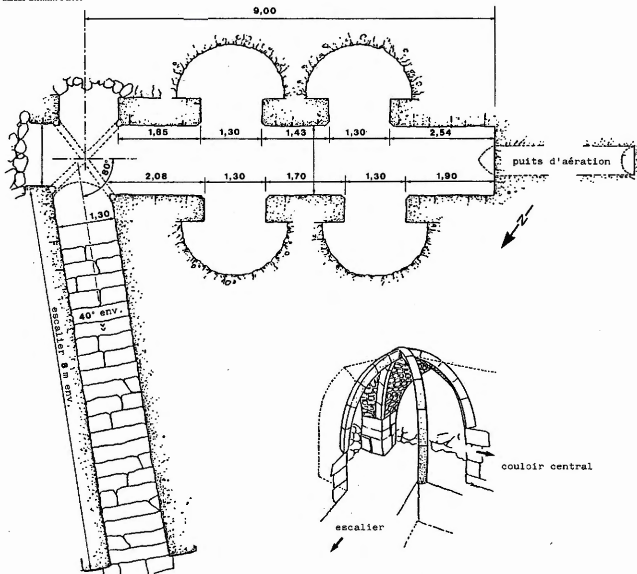
Fig. 1. — Plan de la cave de l'ancienne commanderie des Templiers de Beauvais-en-Gâtinais à Grez-sur-Loing.
